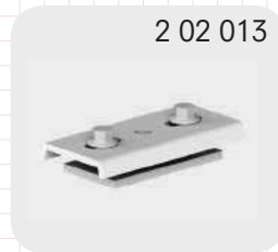
Kapak alt mil menteşe sabitleyicisi x 1 Bottom door pivot hinge fixer x 1 Закрепитель оси нижней дверной петли x 1
